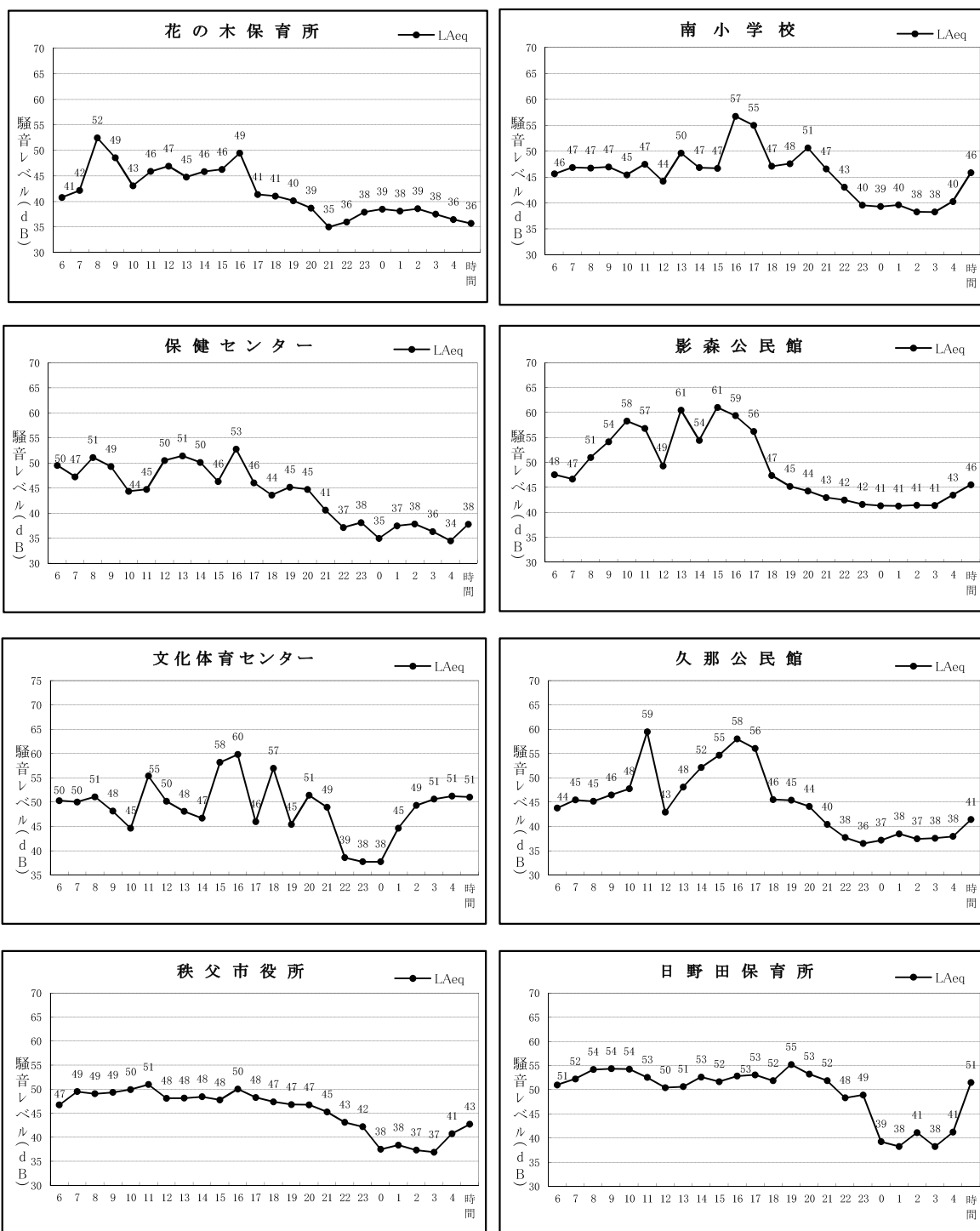
図5-2 平成26年度環境騒音測定結果経時変化図
