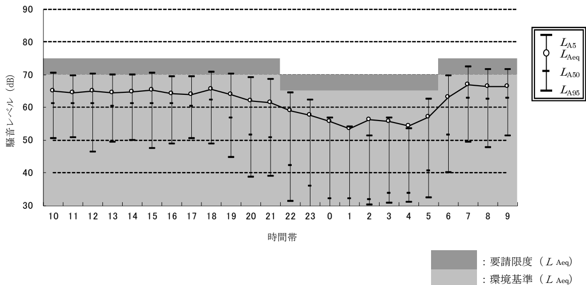
図 3.5.1 騒音時間変化グラフ (2)
