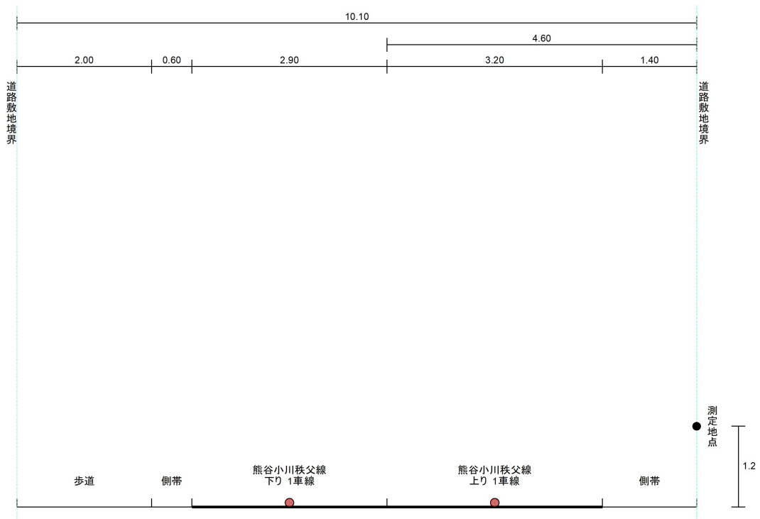
図 3.3.1 調査位置詳細図 (1)
