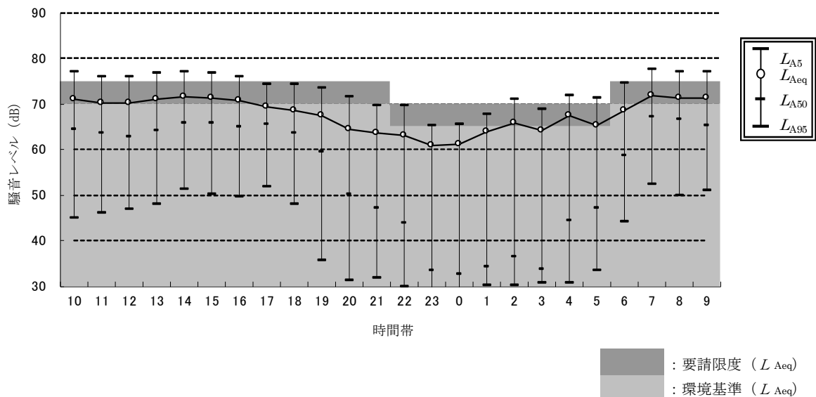
図 3.5.1 騒音時間変化グラフ (1)
