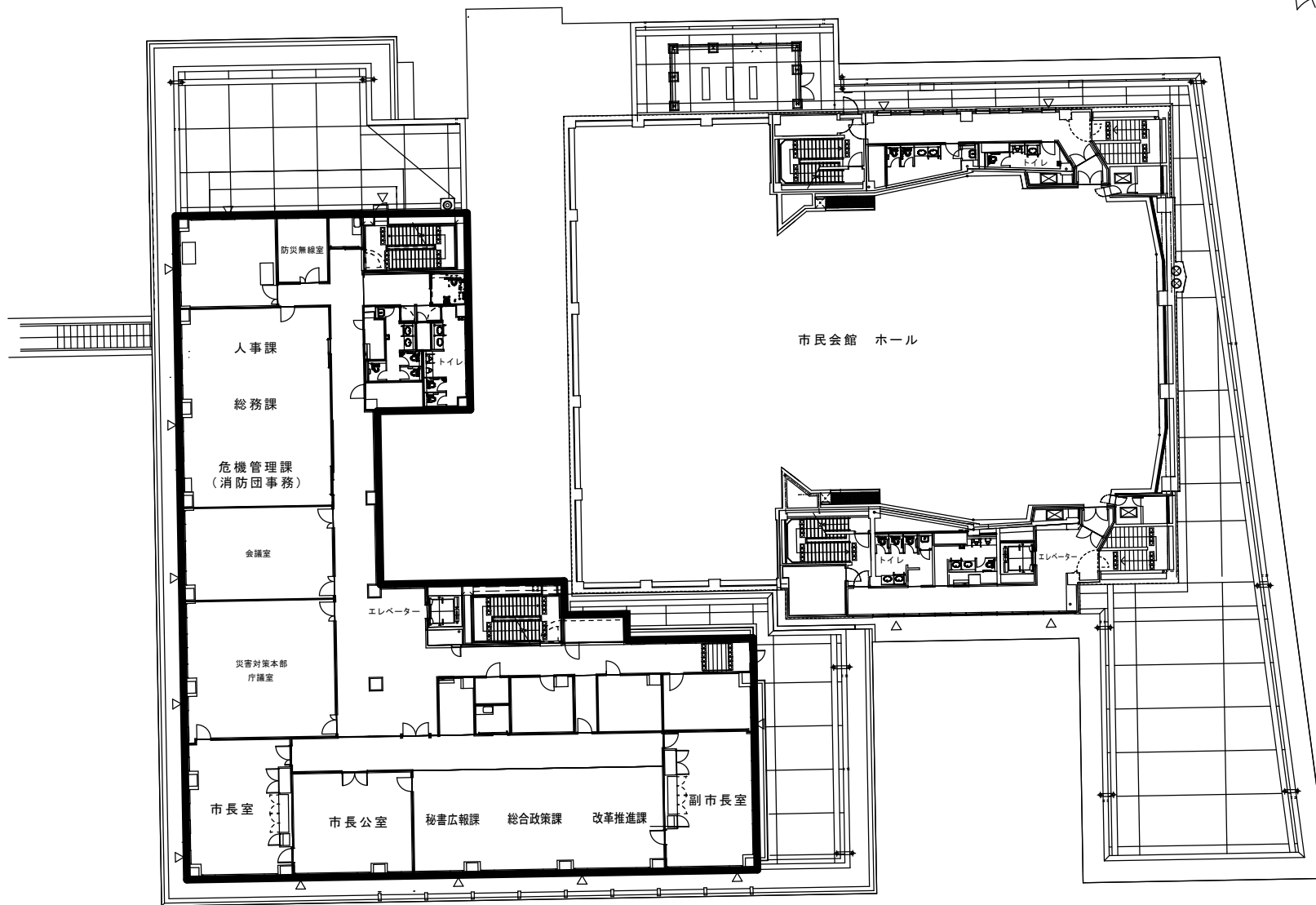
本庁舎・市民会館 3階配置図
