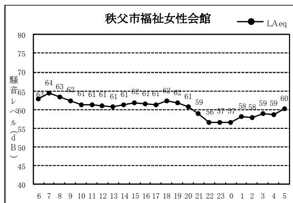
図 3③-4 2020(令和2)年度自動車交通騒音調査結果経時変化
