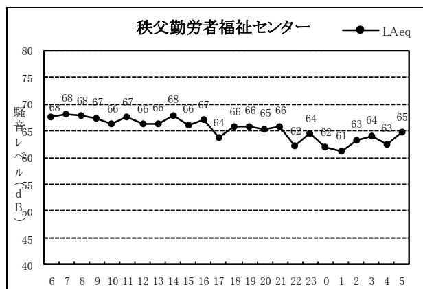
図 3③-4 2020(令和2)年度自動車交通騒音調査結果経時変化
