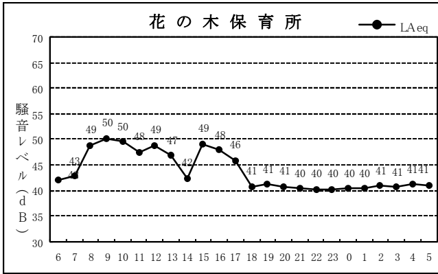
図3③-3 2020（令和2）年度環境騒音測定結果経時変化
