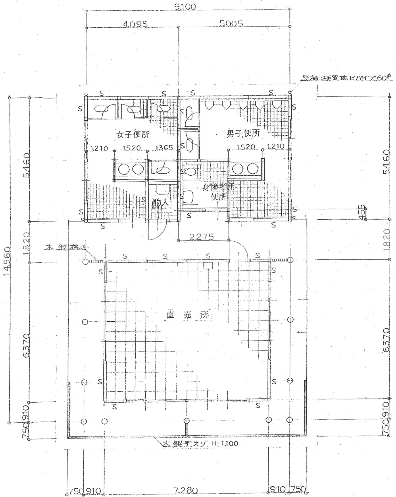
平面図 1:100
